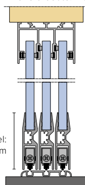
3-sporig Profielbreedte: 7 cm
