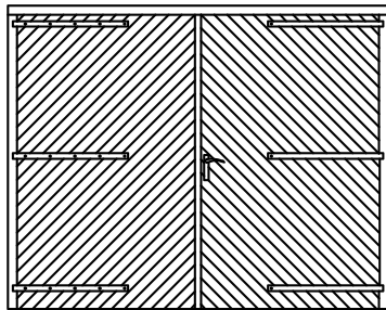
WG02 2290X 2000 (openslaand)
